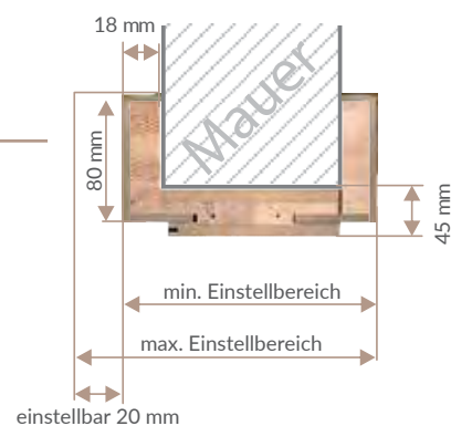
einstellbare Zargen
