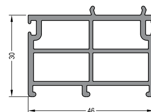
Wärmedämmensatz für Aluschwelle
